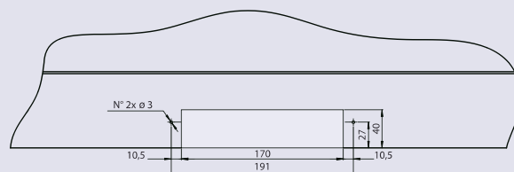
SZEMÉTLAPÁT ADAPTER RÖGZÍTÉSI MÉRETEK
